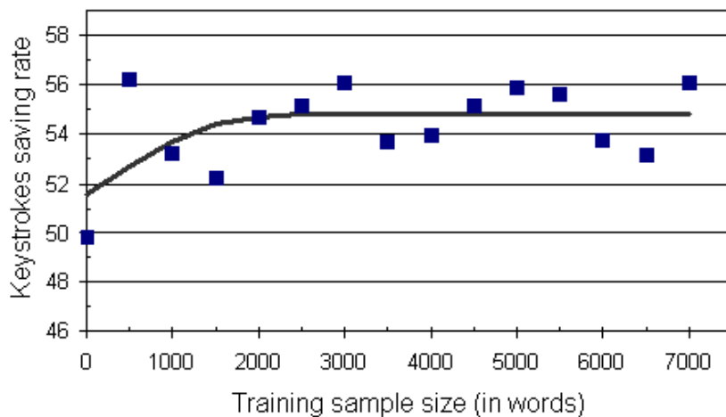
Figure 4. Evolution du taux d'économie de saisies en fonction du nombre de mots déjà composés par l'utilisateur (pour 9 propositions). Un plateau apparaît lorsque 2000 mots environ ont été appris par le module d'apprentissage du modèle utilisateur.
