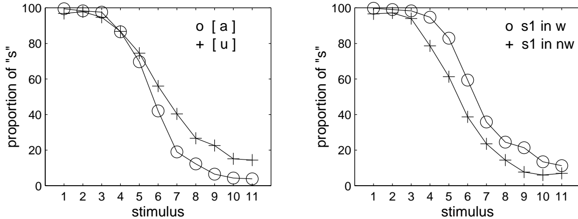
Figure 1: Pourcentages moyens de réponses “s” pour chacune des 11 fricatives sur le continuum [s]-[ʃ]. À gauche: pourcentages décomposés en fonction de la voyelle suivante. À droite: pourcentages décomposés selon le statut lexical de la séquence porteuse. Tiré de Nguyen (1995).
